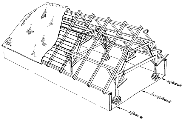
Opengewerkte tekening uit de cursus bouwhistorie
