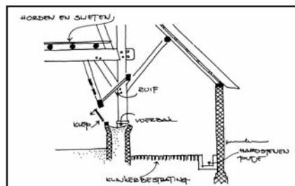
Dwarsdoorsnede van een paardenstal. (Tekening Frank Ruiter).
