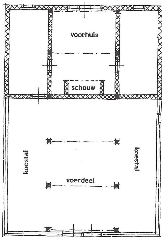
Bedrijfs- en woongedeelte worden gescheiden door de brandmuur.
